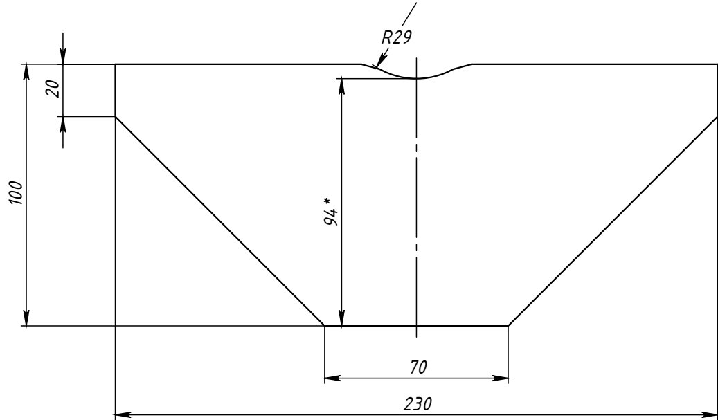
Поз.1 (Корпус) развертка
