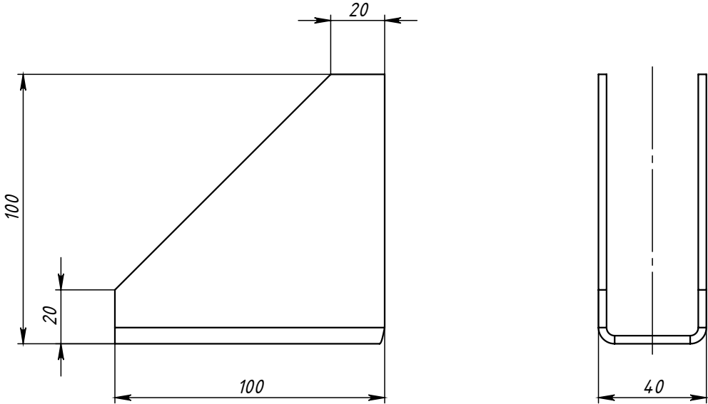
Поз.1 (Корпус)
